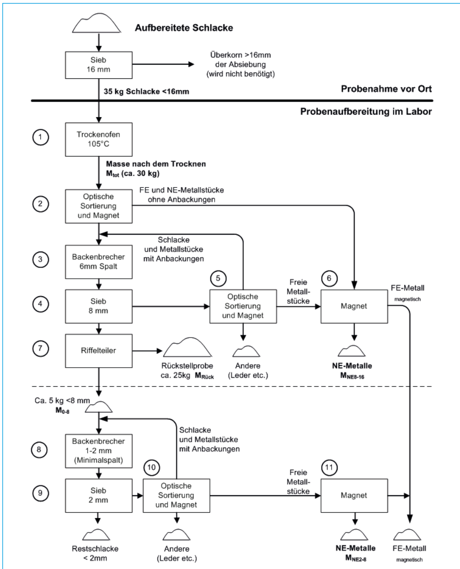
Bild 7: Bestimmung der Gehalte an gediegenen Metallstücken im Rückstand von aufbereiteter MVA-Schlacke gemäß UMTEC-Methode
